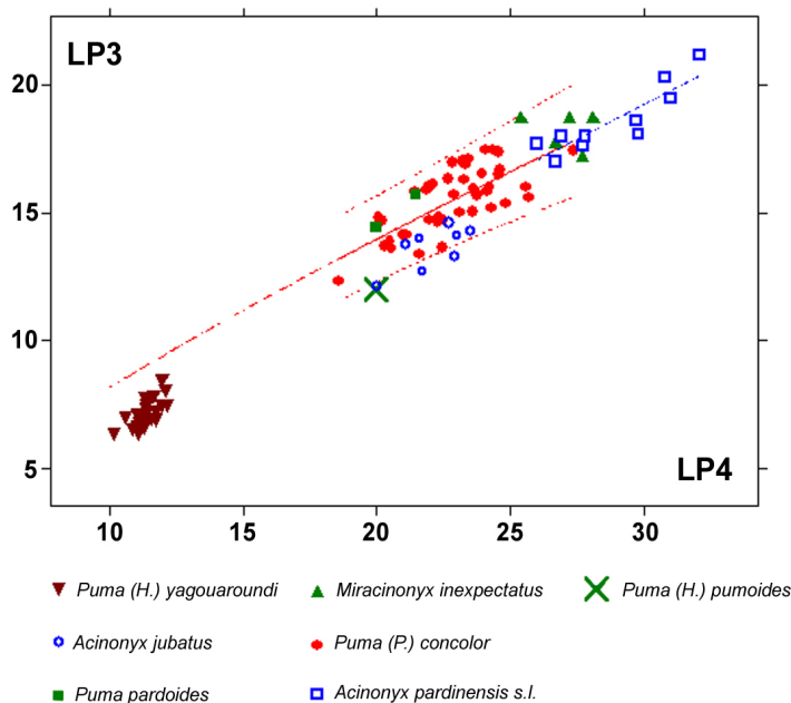
Figura 14. Análisis de dispersión entre la longitud del premolar tercero (LP3) y la longitud del premolar cuarto (LP4). Referencias: líneas continua, Puma (Puma) concolor en forma de curva de potencia ( LP3 = 1.363 \times LP4^{0.777} ); línea discontinua con intervalos cortos, 95% de límite de confianza de P. (P.) concolor ; línea discontinua con intervalos largos, extrapolación al rango de P. (Herpailurus) yagouaroundi . Las medidas utilizadas para P. (P.) concolor , P. (H.) yagouaroundi , P. (H.) pumoides y Acinonyx jubatus se basan en este trabajo; para P. (Viretailurus) pardoides de Hemmer et al. , (2004); para P. (Miracinonyx) inexpectata de Kurtén (1976) y Van Valkenburgh et al. , (1990); y para A. pardinensis s.l. de este trabajo y de varias referencias (Ficcarelli, 1984, Geraads 1997, Hemmer 2001, Qiu et al. , 2004). / Figure 14. Scatter plot P3 length (LP3) against P4 length (LP4). References: continuous line, Puma (Puma) concolor power curve fit ( LP3 = 1.363 \times LP4^{0.777} ); short dashed lines, 95% confidence limit of P. (P.) concolor ; long dashed line, extrapolation to the P. (Herpailurus) yagouaroundi range. The measurements used for P. (P.) concolor , P. (H.) yagouaroundi , P. (H.) pumoides and Acinonyx jubatus is based in this work; for P. (Viretailurus) pardoides from Hemmer et al. , (2004); for P. (Miracinonyx) inexpectata from Kurtén (1976) and Van Valkenburgh et al. , (1990); and for A. pardinensis s.l. from this work and several references (Ficcarelli, 1984, Geraads 1997, Hemmer 2001, Qiu et al. , 2004).
